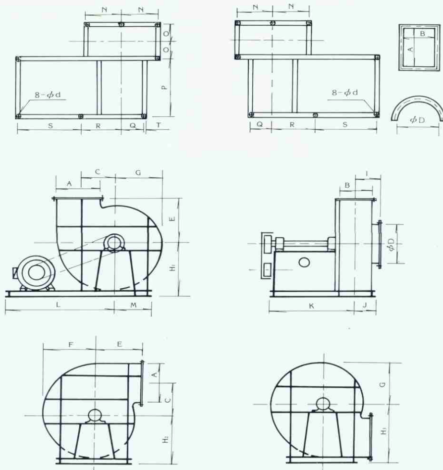
尺寸表 Dimensions
