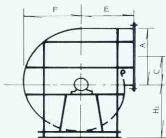
尺寸表 Dimensions
