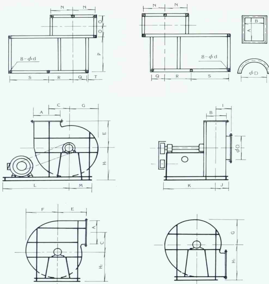
尺寸表 Dimensions
